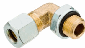
COD:21070412MO COTOVELO MACHO 04MM X M12 COMPLETO
