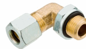
COD:21070612CO COTOVELO MACHO 06MM X M12 COMPLETO
